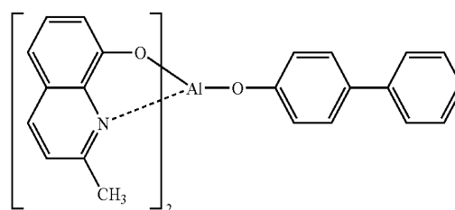
Balq 2:
