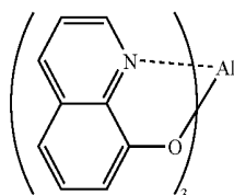
Alq:
